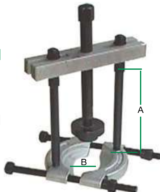
Tirante laterale mm 240 141 287
